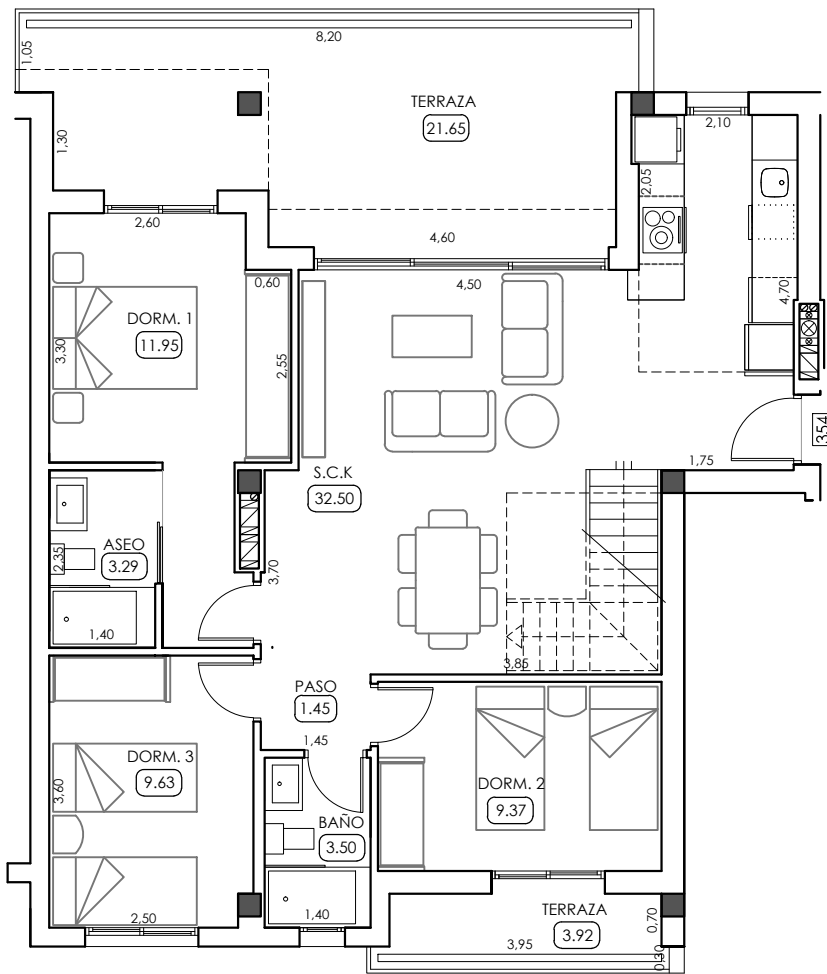
BLOQUE III - PLANO DISTRIBUCIÓN E:1/100
